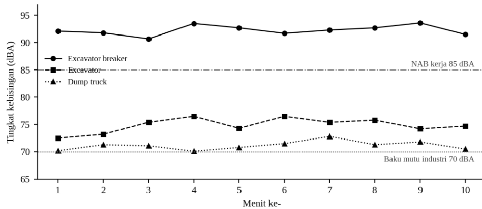
Gambar 3. Tingkat Kebisingan Setiap Menit pada Jarak 2 m dari Sumber
