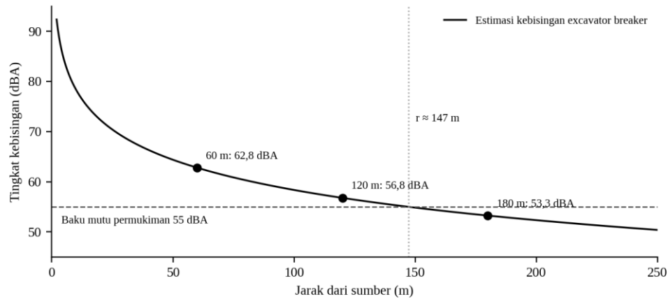
Gambar 4. Estimasi Penurunan Tingkat Kebisingan Excavator Breaker terhadap Jarak
